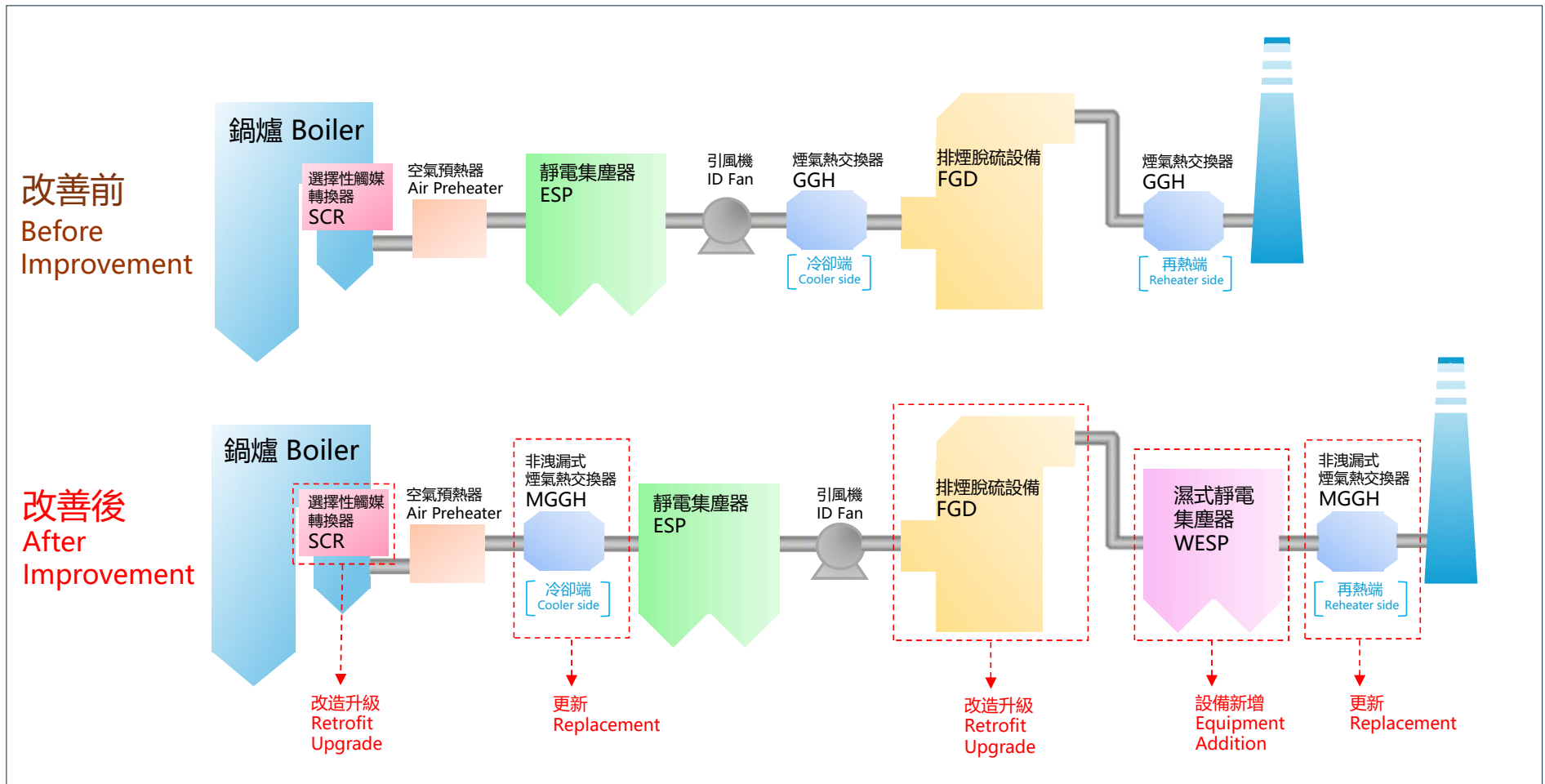
台中發電廠第5至第10機組空污防制設備改善前後比較
